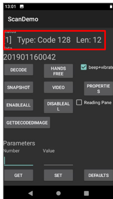
Рисунок 4. Утилита ScanDemo
