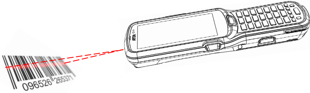
Рисунок 3. Сканирование ШК
